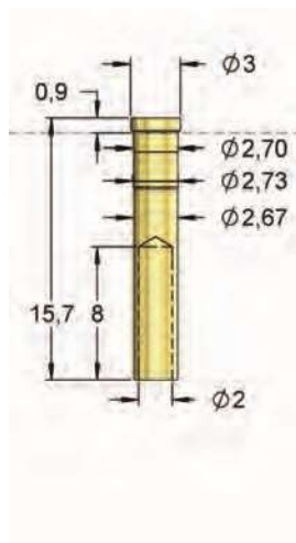
I-P16LA/0.9 30,0 Ampères
