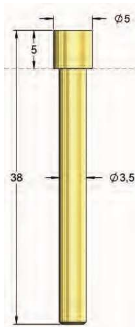
I-P1S2 40,0 Ampères
