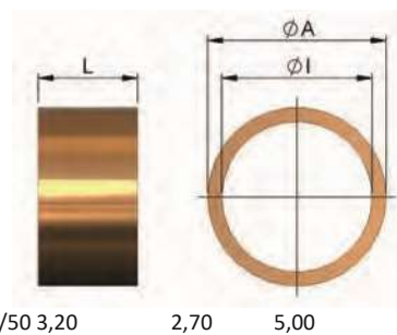
H773DS/50 3,20 2,70 5,00
