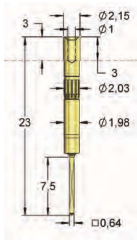
I-D23WW/3 10,0 Ampères
