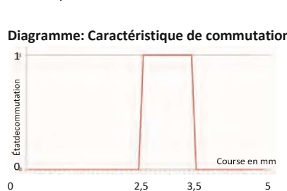
Pointes switch avec fonction Off-On-Off - 2 points de commutation Diagramme: Caractéristique de commutation
