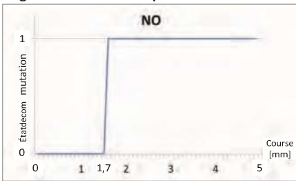
Diagramme: Caractéristique de commutation
