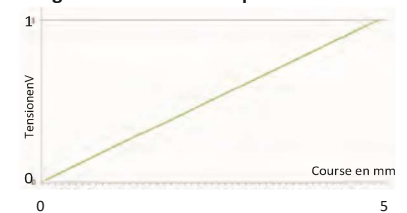
Constante mesure de déplacement Diagramme: caractéristique de mesure
