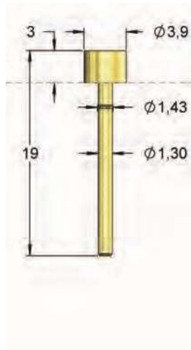
I-D23WW/3 10,0 Ampères
