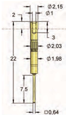
I-D22WW/2 10,0 Ampères
