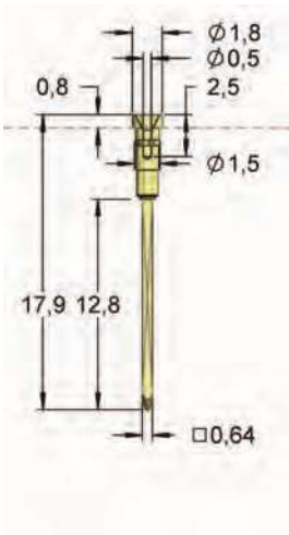
I-C22WW/2 10,0 Ampères
