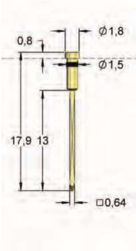
I-Z1 10,0 Ampères
