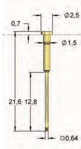
I-P1S4 10,0 Ampères
