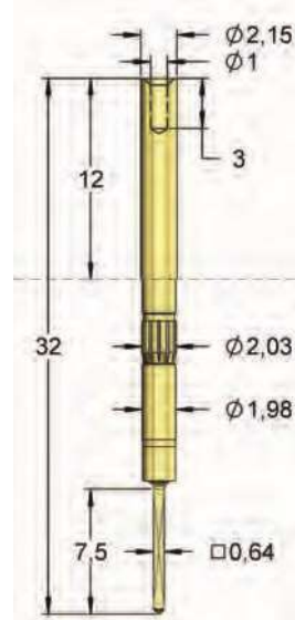
I-D32WW/12 10,0 Ampères
