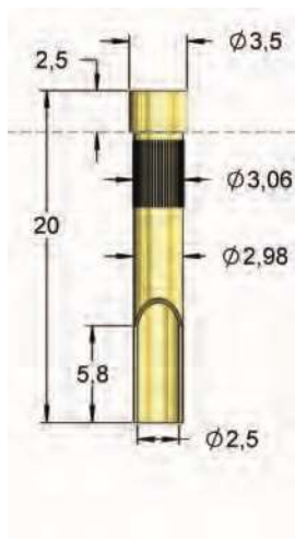
I-P20LA/2.5 30,0 Ampères
