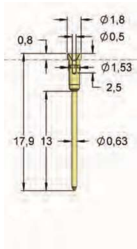
I-D22WW/2 10,0 Ampères
