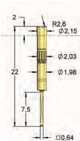
I-C22WW/2 10,0 Ampères
