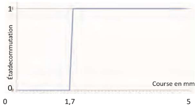
Diagramme: Caractéristique de commutation
