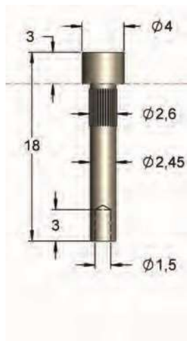
I-P1 30,0 Ampères
