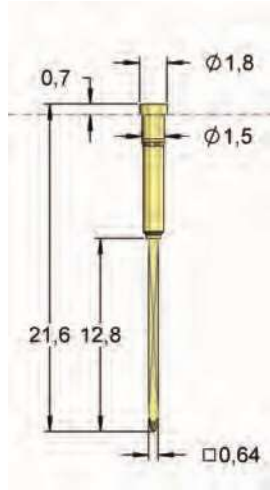
I-Z1WR/0.8 10,0 Ampères
